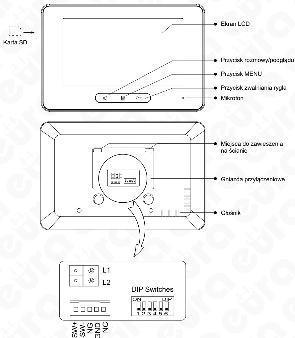
Rys. 3. Widok zewnętrzny monitora VDA-28A5 v.2
